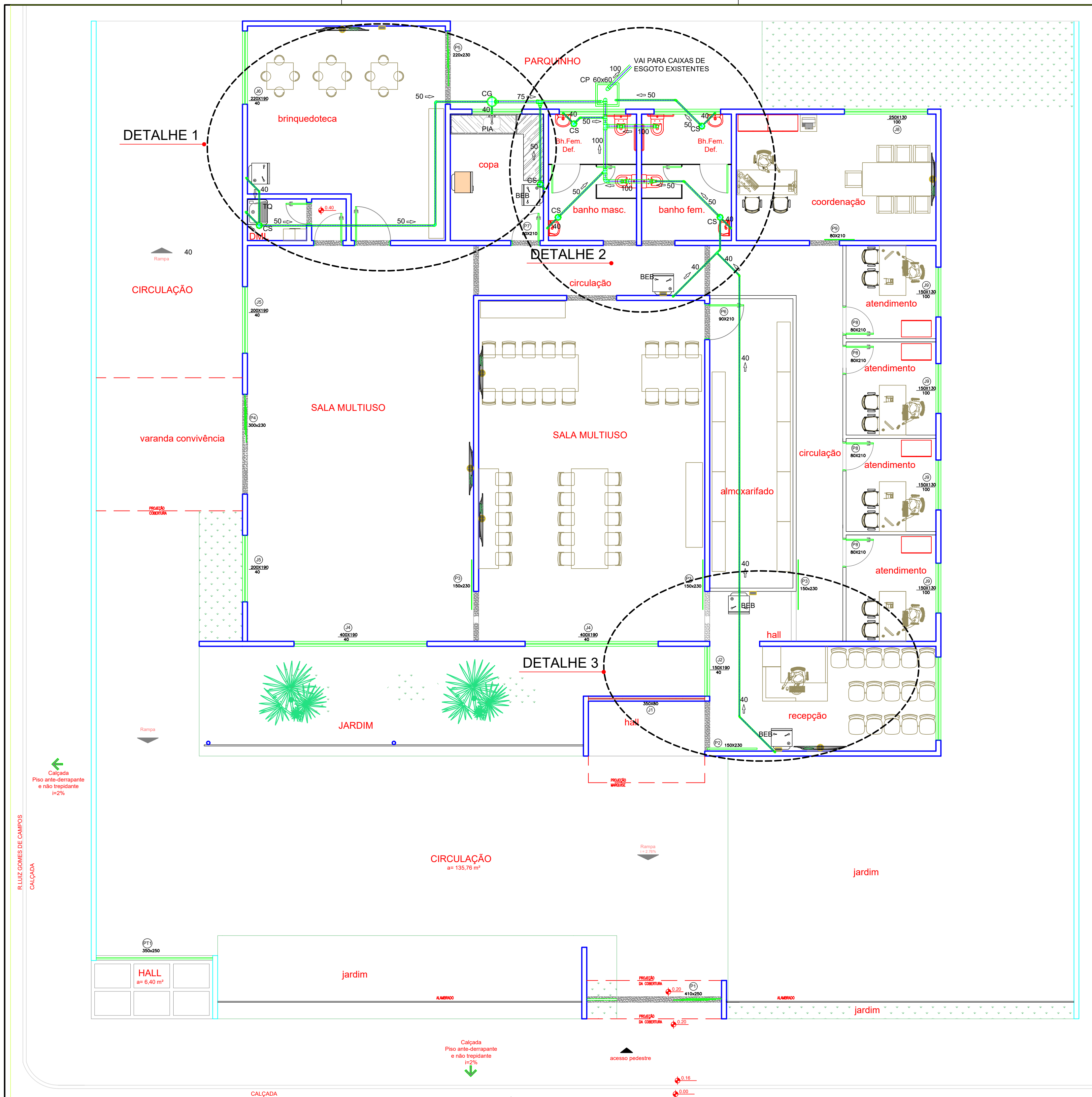
Planta de distribuição de Esgoto Sanitário Escala 1/75
